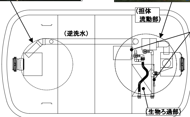
担体流動 生物ろ過槽担体
