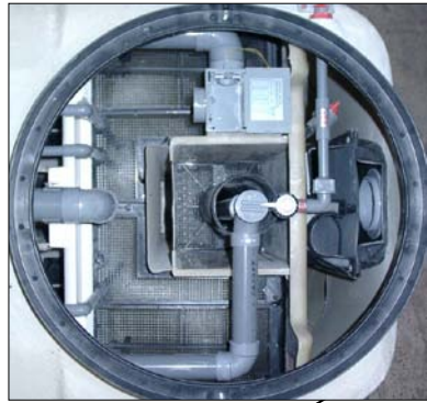
担体流動槽
