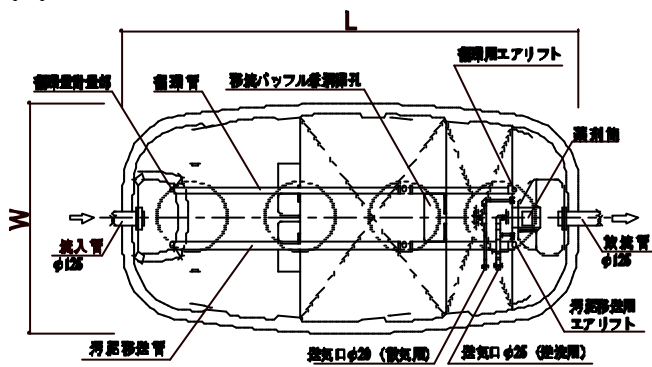
平断面図
