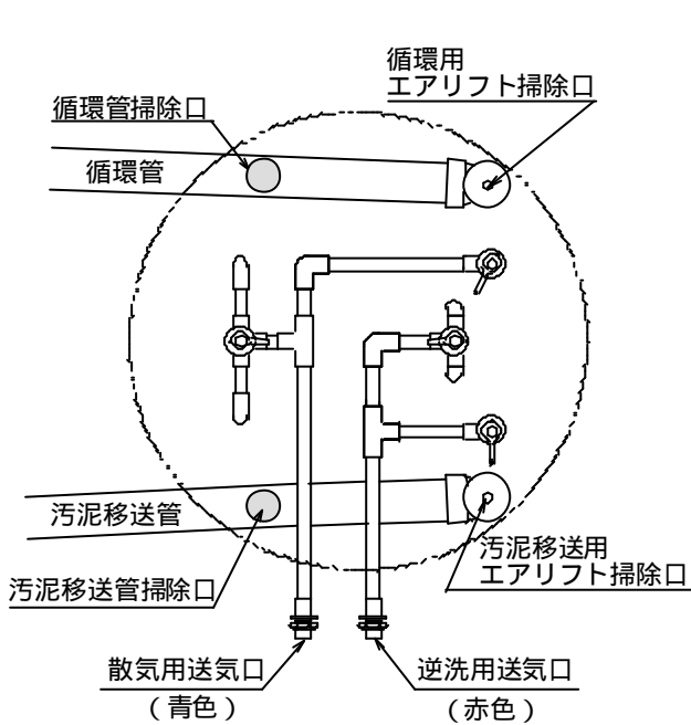
CS型空気配管図
