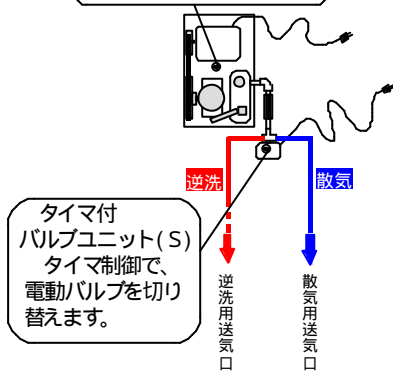
散気・逆洗用ブロワ
