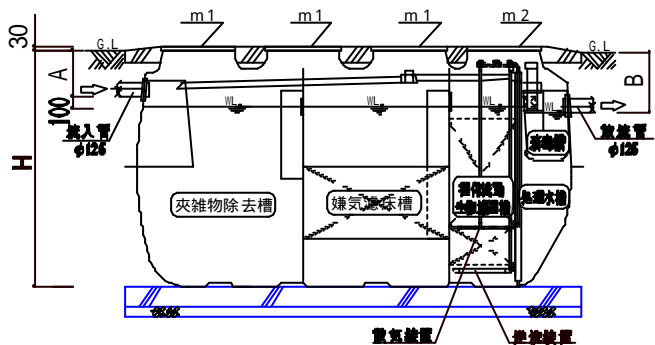
縦断面図
