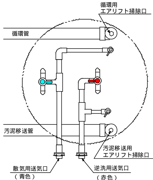
CSL型空気配管図
