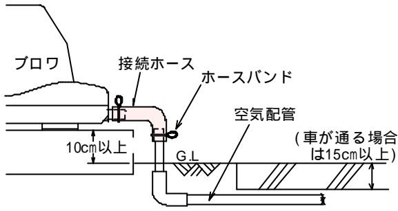
CS 型の設置例
