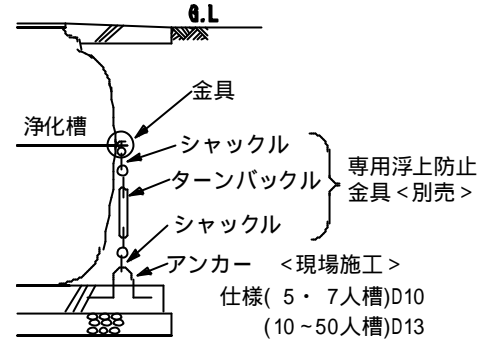
浮上防止金具施工例
