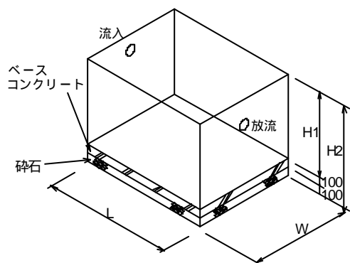
< CS型歩行者荷重の施工例 >
