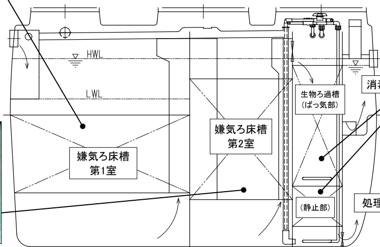
※写真・図は5人槽
