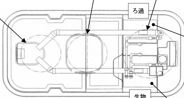
ろ過部担体
