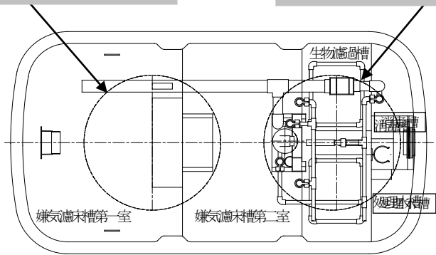
写真・図は5人槽
