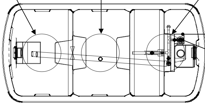
嫌気ろ床槽 第1室ろ材
