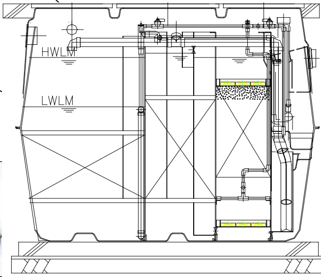
嫌気ろ床槽第2室
